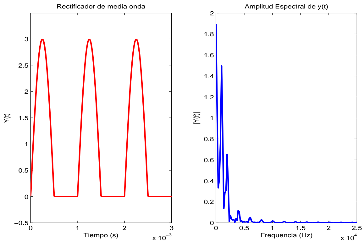
Figure 1: Rectificador de media onda .
