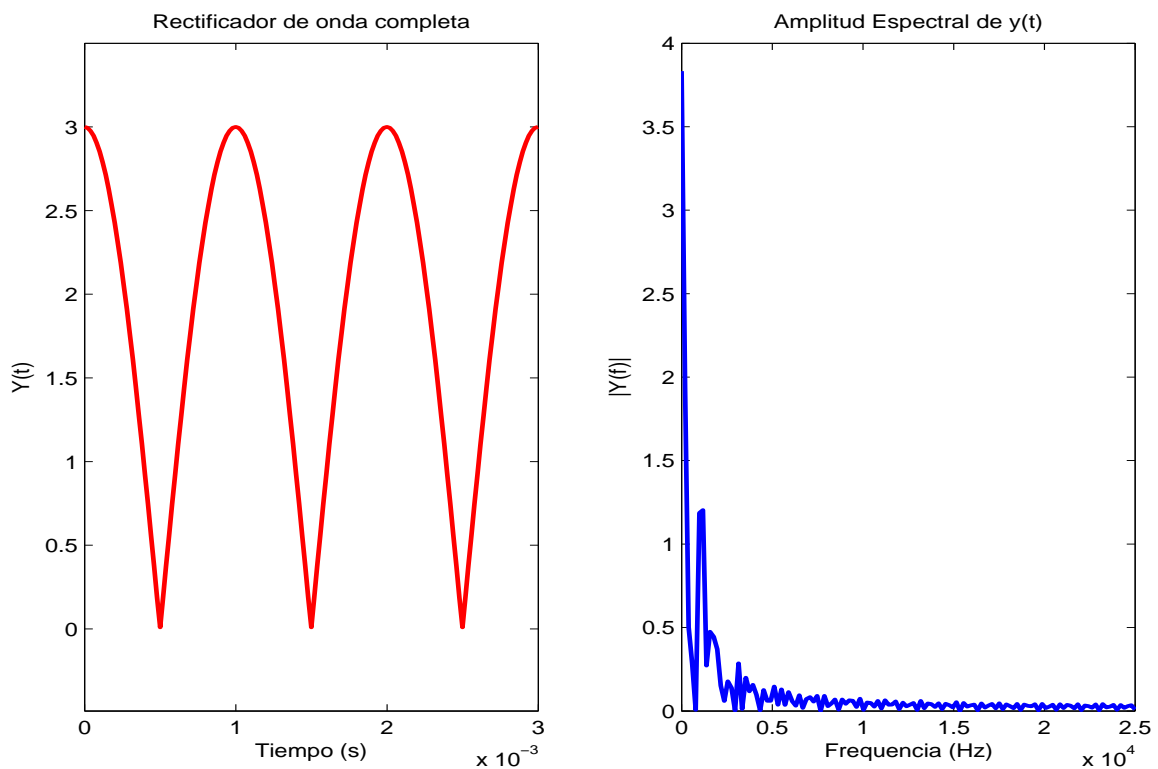
Figure 2: Rectificador de onda completa.
