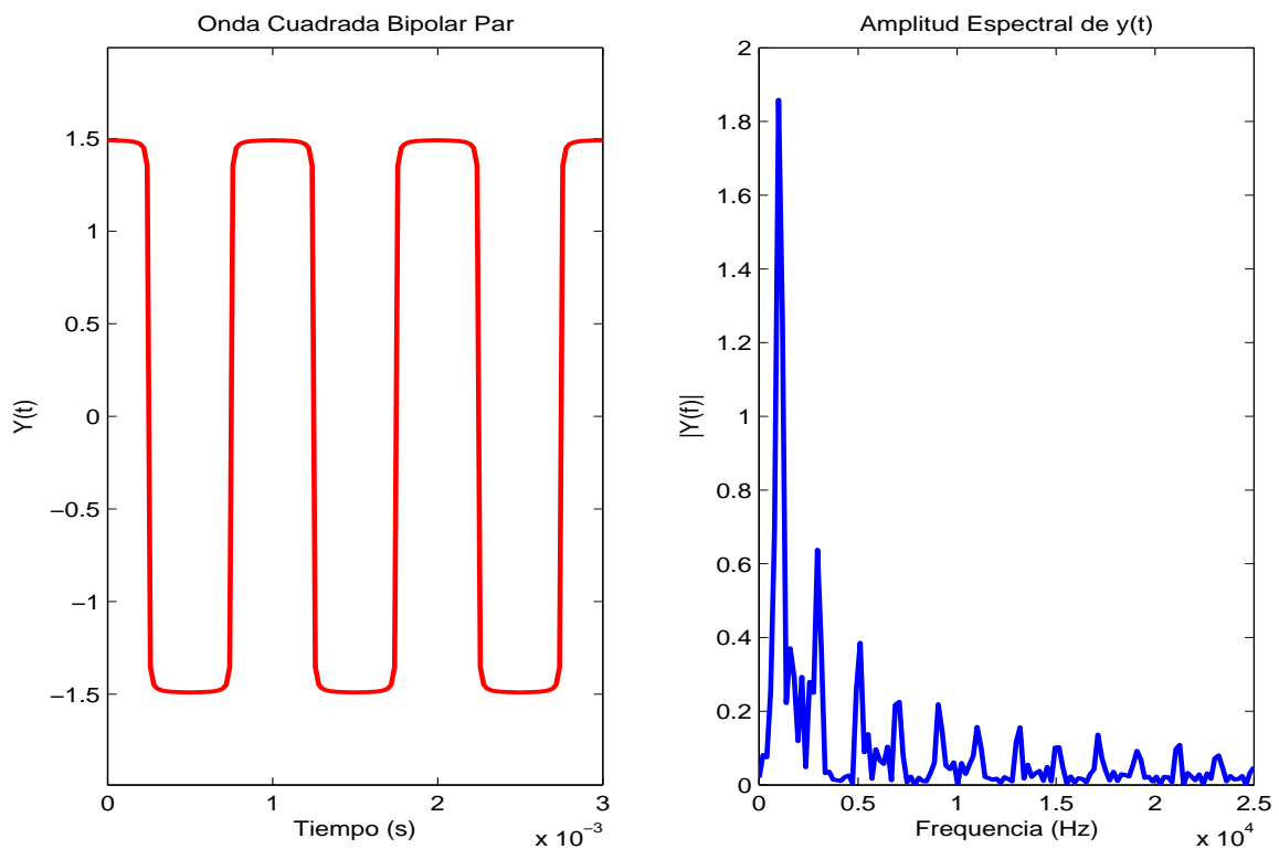
Figure 4: Onda cuadrada bipolar par.
