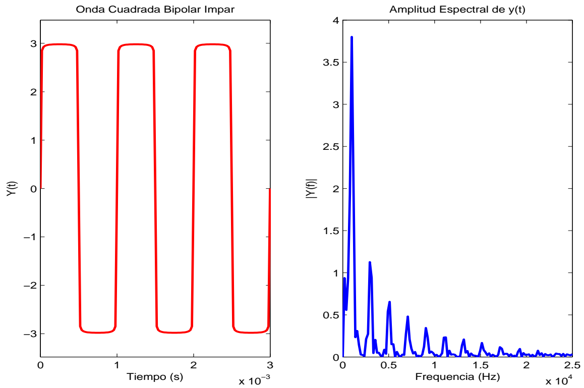
Figure 3: Onda cuadrada bipolar impar.
